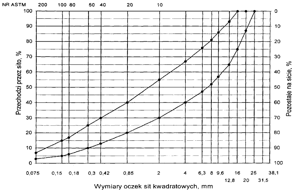
Rys. 4. Krzywe graniczne uziarnienia mieszanki mineralnej BA od 0 do 20 mm do warstwy wiążącej nawierzchni drogi o obciążeniu ruchem KR1 lub KR2
