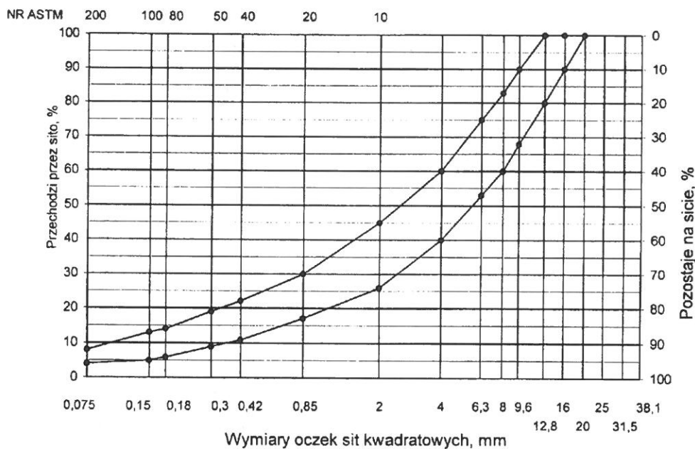
Rys. 1. Krzywe graniczne uziarnienia mieszanki mineralnej BA od 0 do 16 mm do podbudowy nawierzchni drogi o obciążeniu ruchem KR 1 lub KR 2
