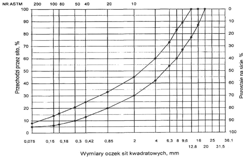
Rys. 4. Krzywe graniczne uziarnienia mieszanki mineralnej BA od 0 do 16 mm do warstwy wyrównawczej nawierzchni drogi o obciążeniu ruchem od KR3 do KR6
