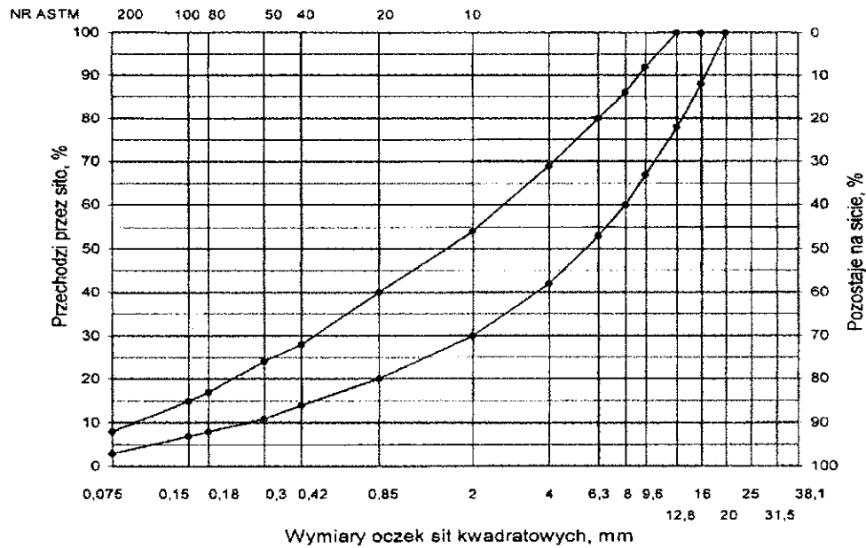
Rys. 5. Krzywe graniczne uziarnienia mieszanki mineralnej BA od 0 do 16 mm do warstwy wiążącej nawierzchni drogi o obciążeniu ruchem KR1 lub KR2
