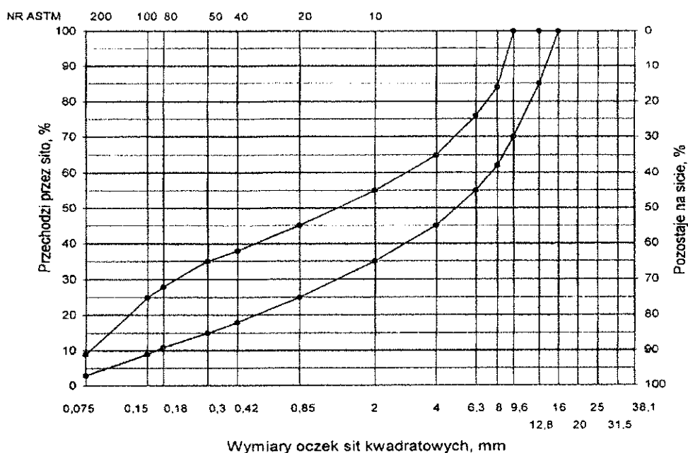
Rys. 6. Krzywe graniczne uziarnienia mieszanki mineralnej BA od 0 do 12,8 mm do warstwy wiążącej nawierzchni drogi o obciążeniu ruchem KR1 lub KR2
